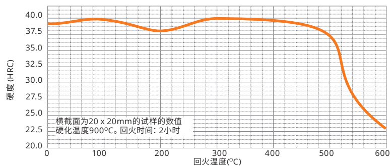
回火曲线
