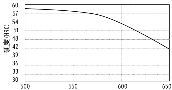
回火曲线图
